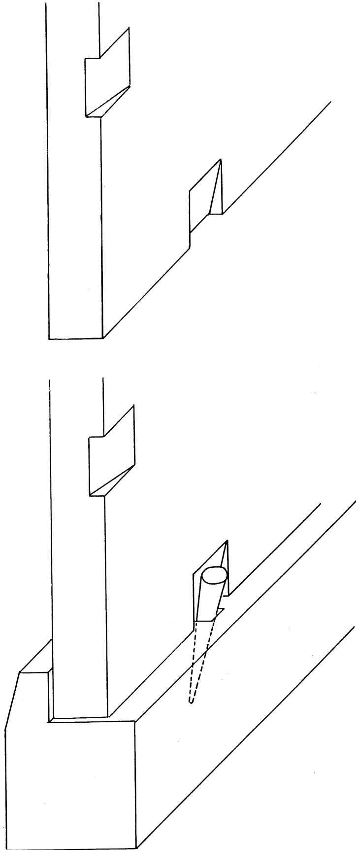
Mögliche Befestigungsform für die Tafel im Schmuckrahmen mit Holznägeln.
