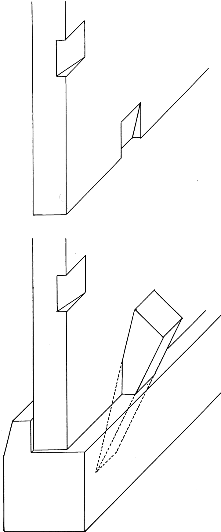
Mögliche Befestigungsform für die Tafel im Schmuckrahmen mit Keilen.
